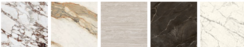
KM12 Breccia
